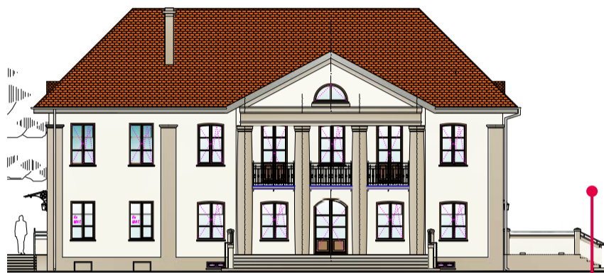
ELEWACJA ZACHODNIA
